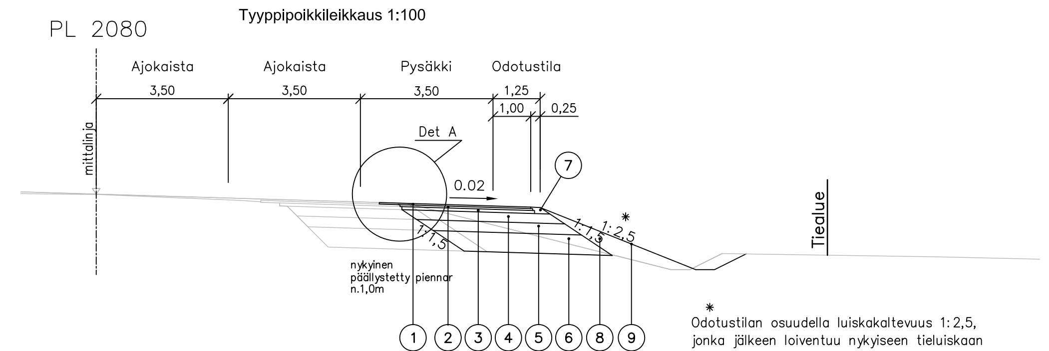
Vt13 raskaanliikenteen odotuskaistan rakennussuunnitelman mukainen rakenne
