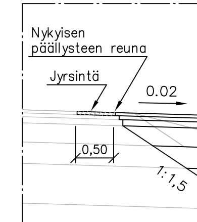
Det A 1:50
