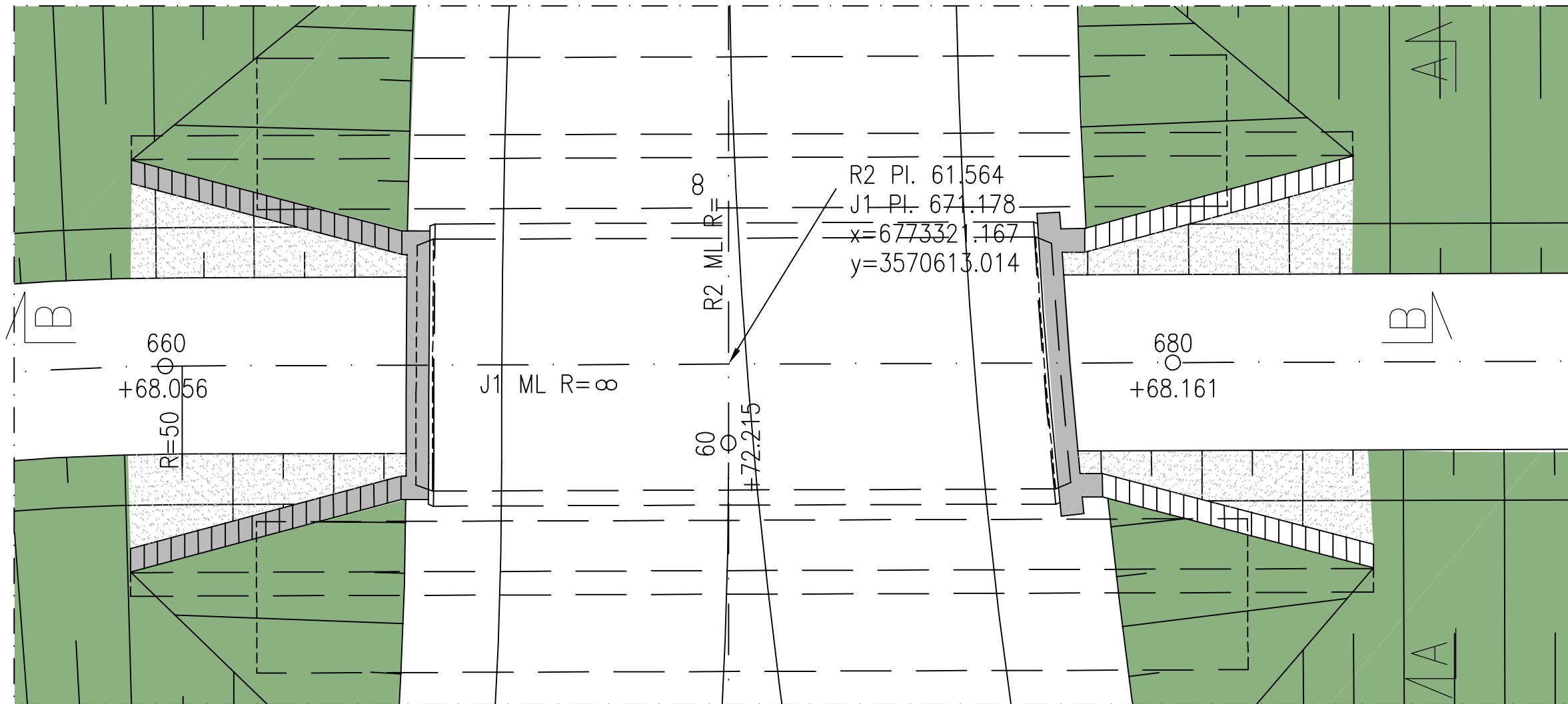
TASOKUVA 1:100
