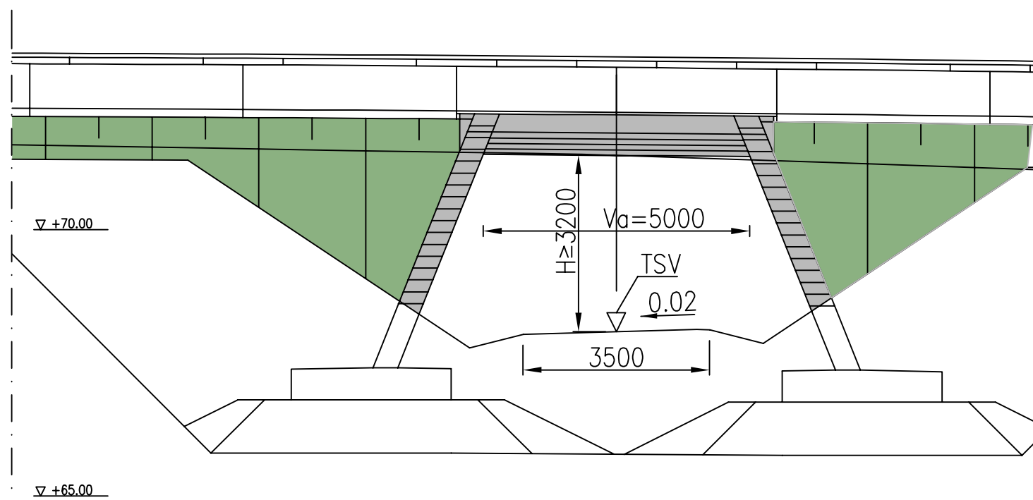
TASOKUVA 1:100
